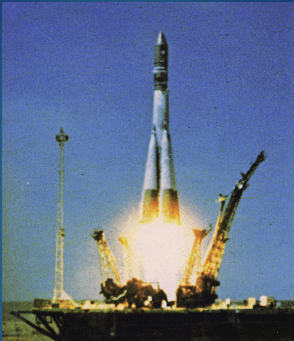
Старт космического корабля «Восток» («Восток-1»)
