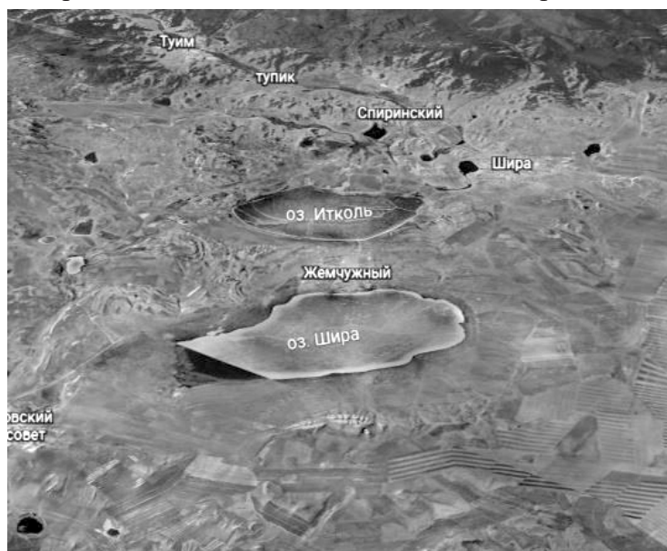
Рис. 1. Стулообразный рельеф.
